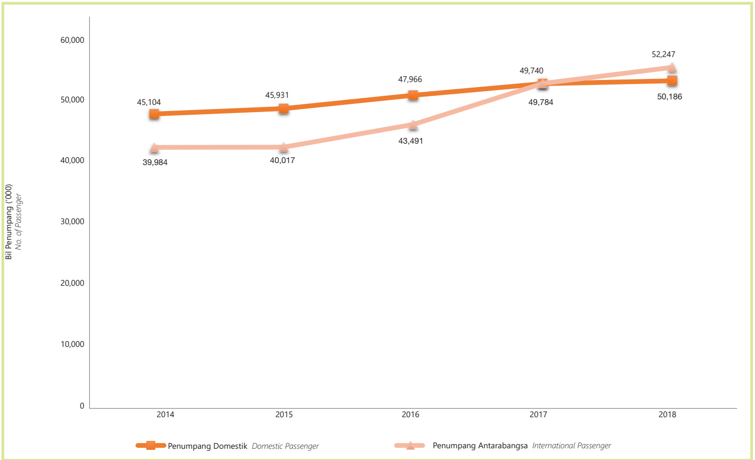
Carta 4. 1: JUMLAH PENUMPANG DOMESTIK DAN ANTARABANGSA YANG DIKENDALIKAN DI LAPANGAN TERBANG, MALAYSIA, 2014-2018 Chart 4.1: Total Number of Domestic and International Passengers Handled by Airport, Malaysia, 2014-2018
